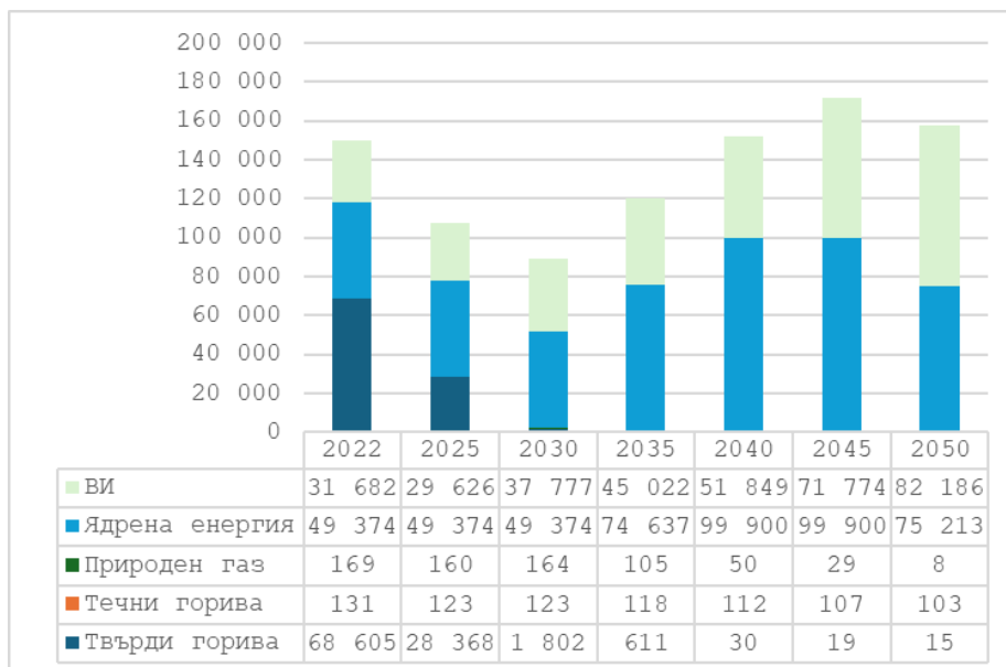
Фигура 15: Производство на първична енергия (GWh), сценарий WAM
