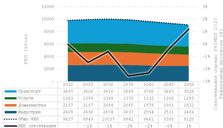
Фигура 64: Крайно енергийно потребление по сектори (ktoe) и спестявания спрямо стойността за съответната година от PRIMES 2020 по сценарий (B)EST WEM
