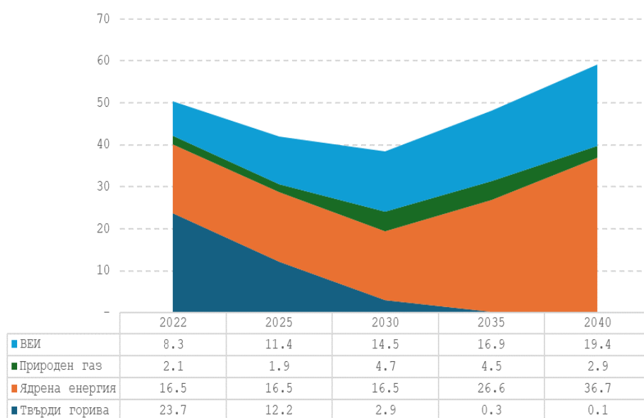
Фигура 77: Бруто производство на електрическа енергия по горива през периода 2022 – 2040 г., GWh, сценарий WEM
