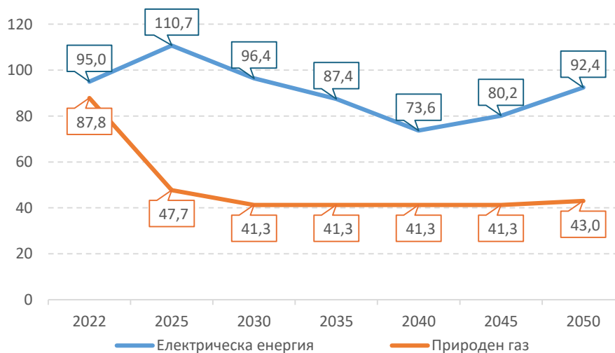
Фигура 96: Потребителски цени на електрическата енергия и природен газ през периода 2022 – 2050 г., EUR '15/MWh, сценарий WEM
