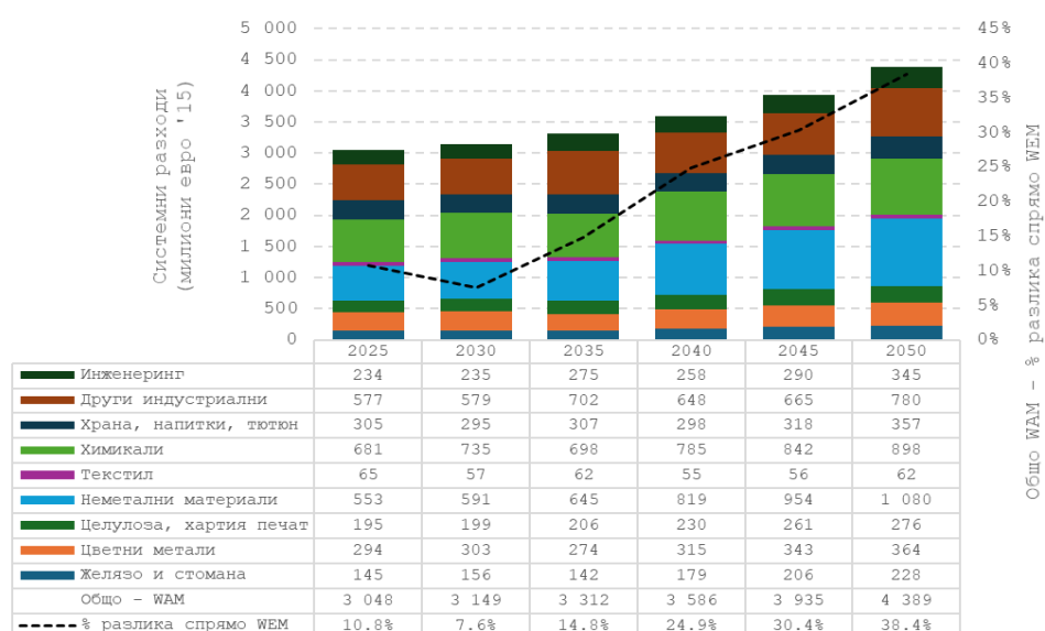
Фигура 104: Системни разходи в индустрията по сектори, (B)EST WAM прогнози (млн. EUR'15)
