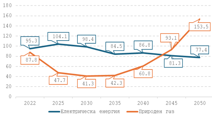
Фигура 19: Потребителски цени на електрическа енергия и природен газ в България, исторически данни (2022 г.) и прогнози (B)EST WAM (2025-2050 г.) (15 EUR/MWh)
