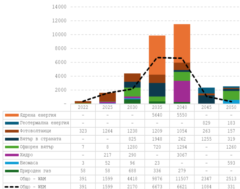
Фигура 23: Инвестиционни разходи за електрическа енергия по видове централи, (B)EST WAM прогнози (млн. евро'15)
