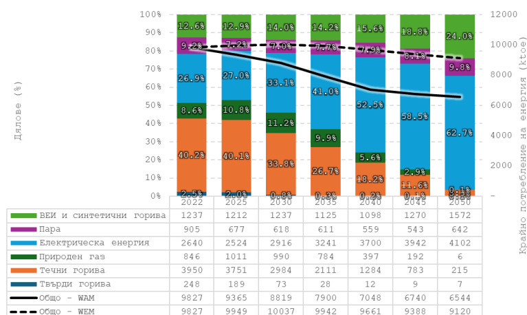
Фигура 106: Крайното потребление на енергия по горива (ktoe) и дялове (%) по сценарий WAM и сравнение WEM и WAM
