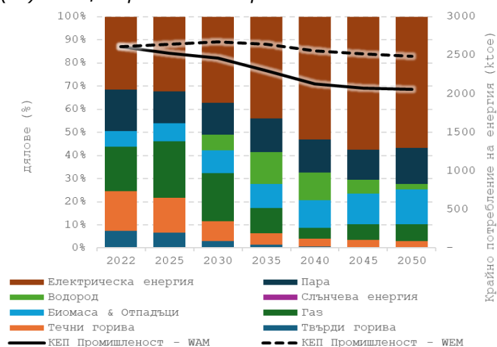
Фигура 108: Крайно потребление на енергия в сектор Индустрия (ktoe) и дялове (%) по сценарий WAM и сравнение WEM и WAM
