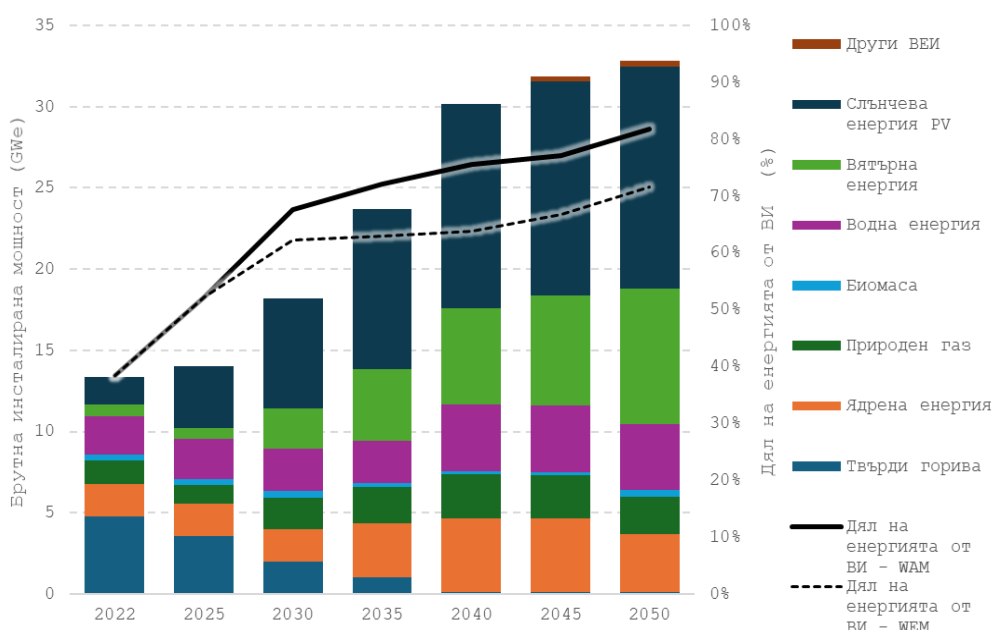
Фигура 114: Брутна инсталирана мощност за производство на ел. енергия по видове централи (GW) и дял на ВИ в брутната инсталирана мощност, сценарий WAM
