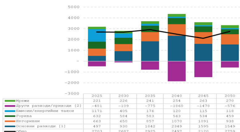
Фигура 97: Разходи за доставка на ел. енергия по категории и общо, (B)EST WEM прогнози (млн. EUR'15)
