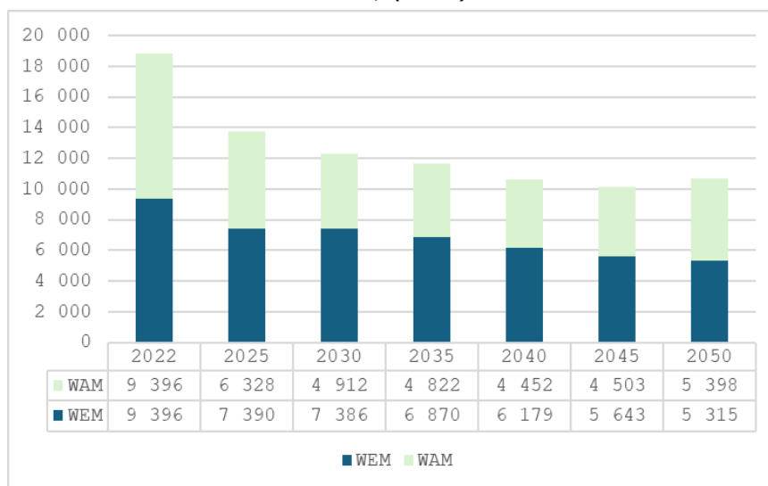
Фигура 119: Сравнение на производство на топлинна енергия по сценарии WEM и WAM, (GWh)
