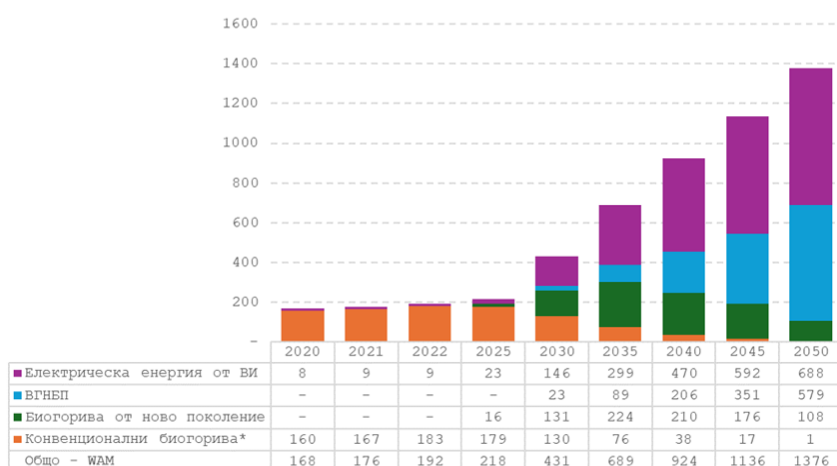
Фигура 10: Прогнозно развитие на възобновяемата енергия в сектор транспорт по видове горива, ktce
