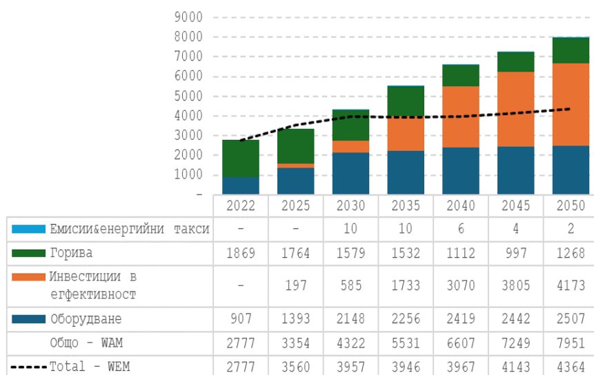
Фигура 21: Системни разходи в домакинствата по категории в България, (B)EST WAM прогнози (млн. евро'15)
