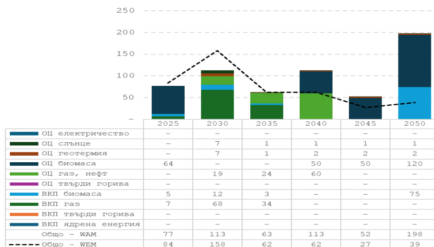
Фигура 24: Инвестиционни разходи в КИ и ОЦ по видове централи, (B)EST WAM прогнози (млн. евро'15)
