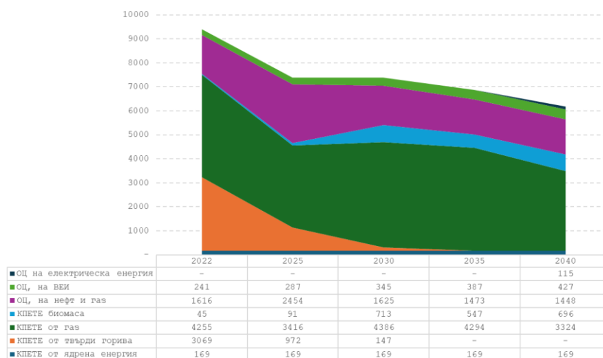
Фигура 80: Производство на топлинна енергия по видове горива през периода 2022 – 2040 г., GWh, сценарий WEM
