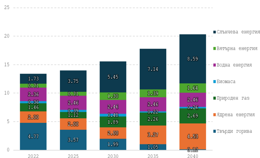
Фигура 91: Инсталирана мощност по видове централи през периода 2022 – 2040 г., GW, Сценарий WEM
