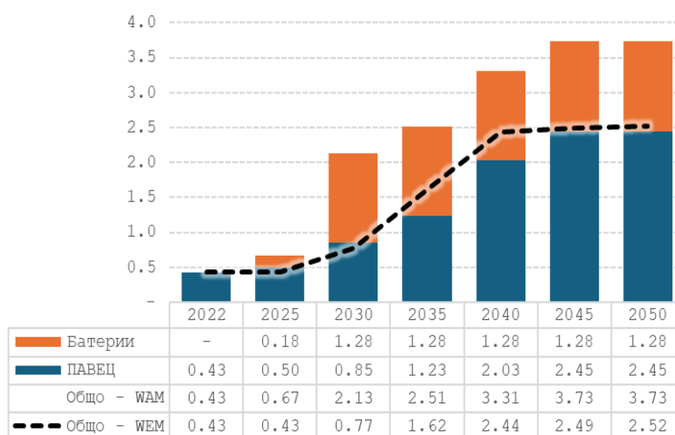
Фигура 117: Инсталирана мощност за съхранение на ел. енергия (GW) в България, исторически данни (2022) и (B)EST WAM прогнози (2025-2050)
