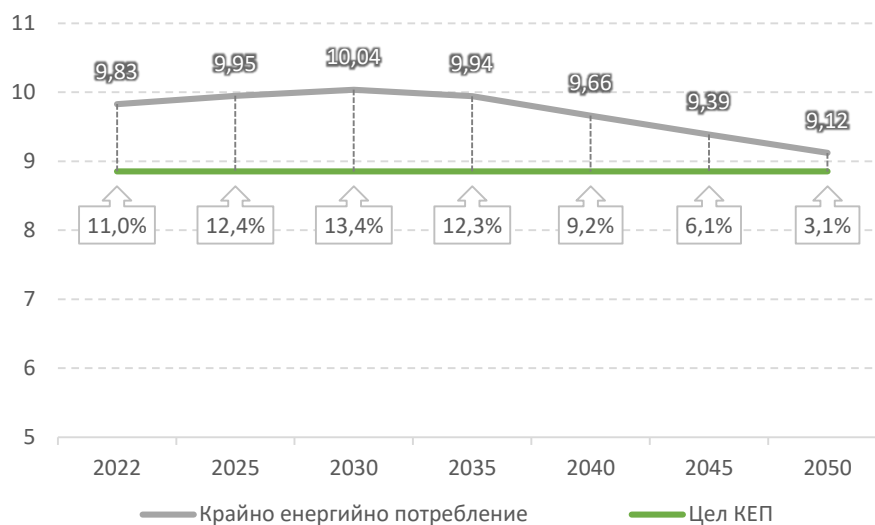
Фигура 63: Крайно потребление на енергия (Mtoe) по сценарий (B)EST WEM
