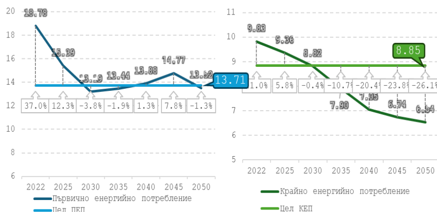
Фигура 17: Първично и крайно потребление на енергия в България, цел, исторически данни (2022 г.) и прогнози (B)EST WAM (2025-2050 г.) (Mtoe)
