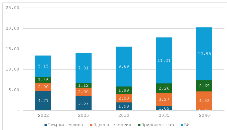
Фигура 92: Инсталирана мощност по видове енергоносители през периода 2022 – 2040 г., GW, сценарий WEM
