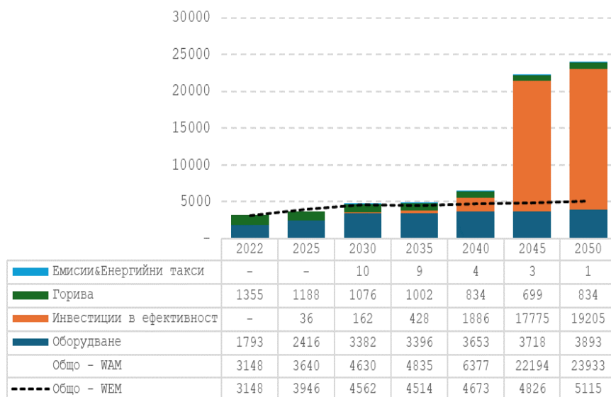
Фигура 22: Системни разходи за услуги и селско стопанство по категории в България, (B)EST WAM прогнози (млн. евро'15)
