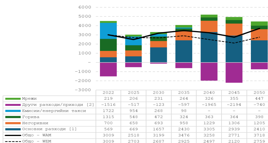
Фигура 25: Разходи за доставка на електрическа енергия, (B)EST WAM прогнози (млн. евро'15)
