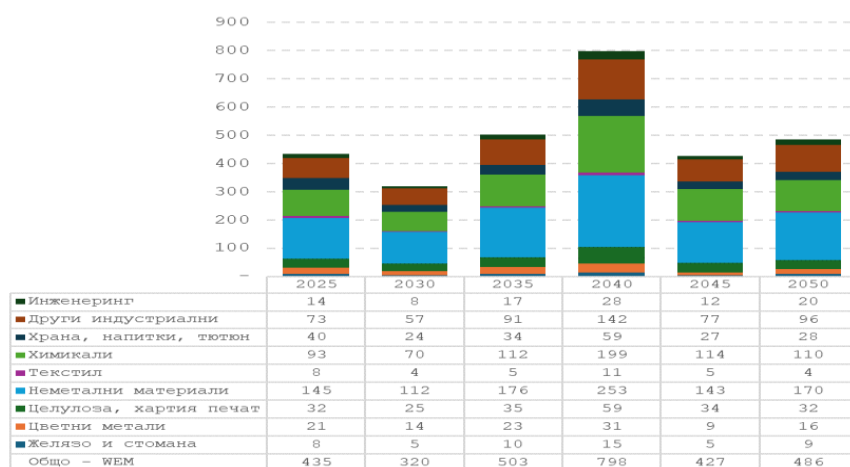
Фигура 120: Инвестиционни разходи за оползотворяване на топлина в индустрията по сектори, (B)EST WEM прогнози (млн. EUR'15 за 5 годишен период)
