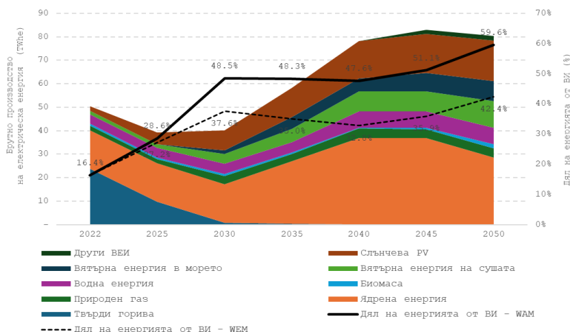
Фигура 112: Брутно производство на електрическа енергия по видове централи (TWh) и дял на ВИ (%), исторически данни (2022) и (B)EST WAM прогнози (2025-2050)
