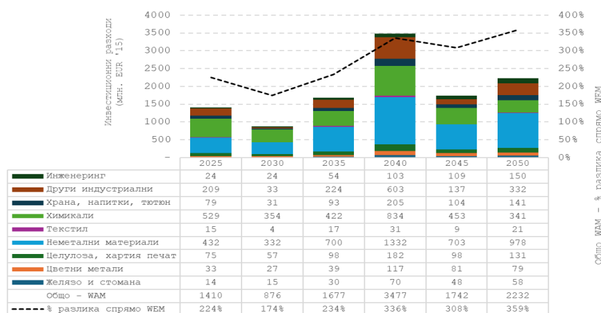
Фигура 20: Инвестиционни разходи за оползотворяване на топлина в промишлеността по сектори в България, (B)EST WAM прогнози (млн. EUR '15 за 5 год. период)
