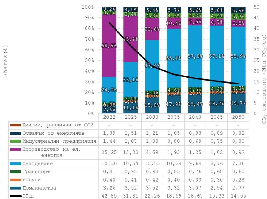
Фигура 47: Емисии на CO 2 в енергетиката по сектори в България исторически данни (2022 г.) и прогнози (B)EST WEM (2025-2050 г.) (Mtn CO 2 -eq)
