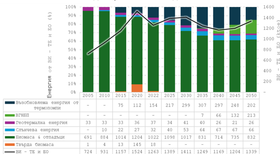
Фигура 9: Енергия от възобновяеми източници в сектор топлинна енергия и енергия за охлаждане, ktoe и по видове ВИ в %
