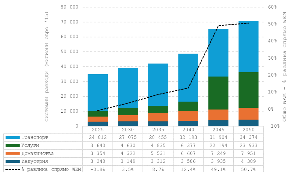
Фигура 103: Общи системни разходи по сектори в България, (B)EST WAM прогнози (милиони евро'15)
