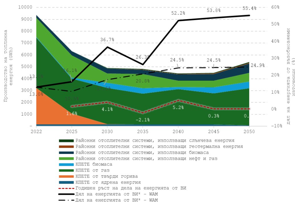
Фигура 118: Производство на топлинна енергия по горива (GWh) и дялове (%) на ВИ в производството на топлинна енергия по сценарий WAM и сравнение на сценариите WEM и WAM
