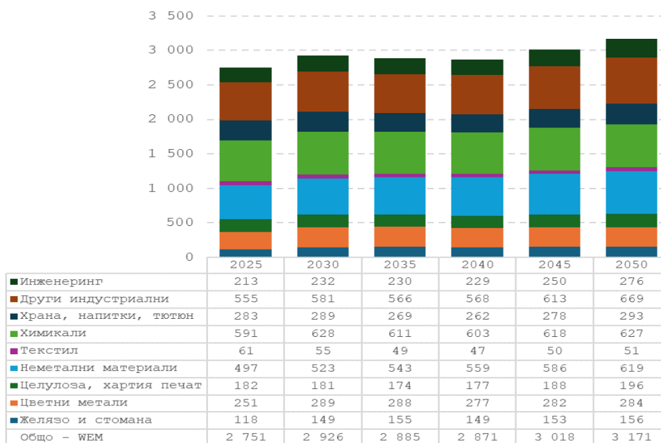
Фигура 95: Системни разходи в индустрията по сектори (директна употреба, вкл. оползотворяване на топлина), (B)EST WEM прогнози (млн. EUR'15)
