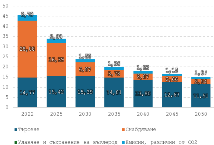
Фигура 46 : Свързани с енергетиката емисии на парникови газове в България исторически данни (2022 г.) и прогнози (B)EST WEM (2025-2050 г.) (Mtn CO 2 -eq)
