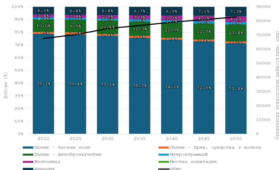
Фигура 37: Пътнически транспорт, исторически данни и прогнози (млн. ркм и дялове в %)
