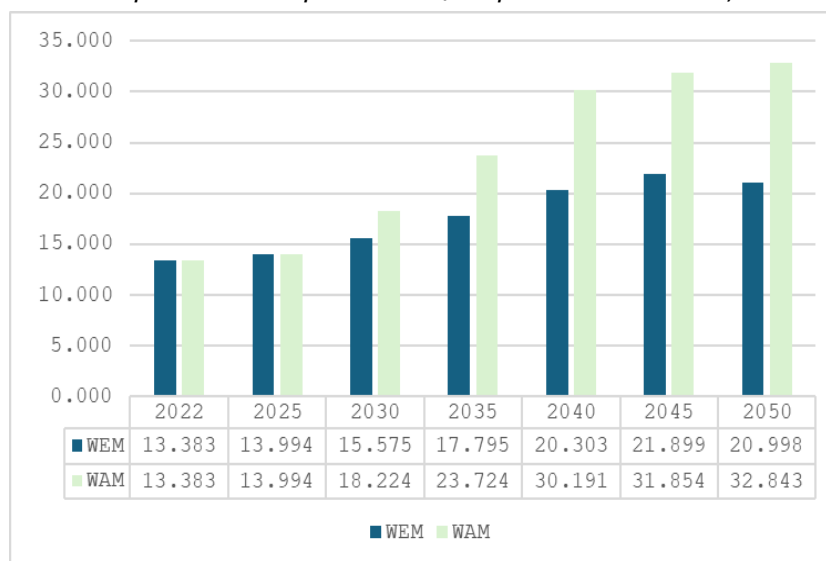
Фигура 115: Сравнение на бутната инсталирана мощност за производство на електрическа енергия по сценарии WEM и WAM, GW
