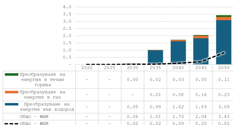
Фигура 116: Инсталирана мощност на централи power-to-X (GW), исторически данни (2022 г.) и (B)EST WAM прогнози (2025-2050 г.) и общ инсталиран капацитет на инсталации power-to-X в (B)EST WEM (2025-2050)
