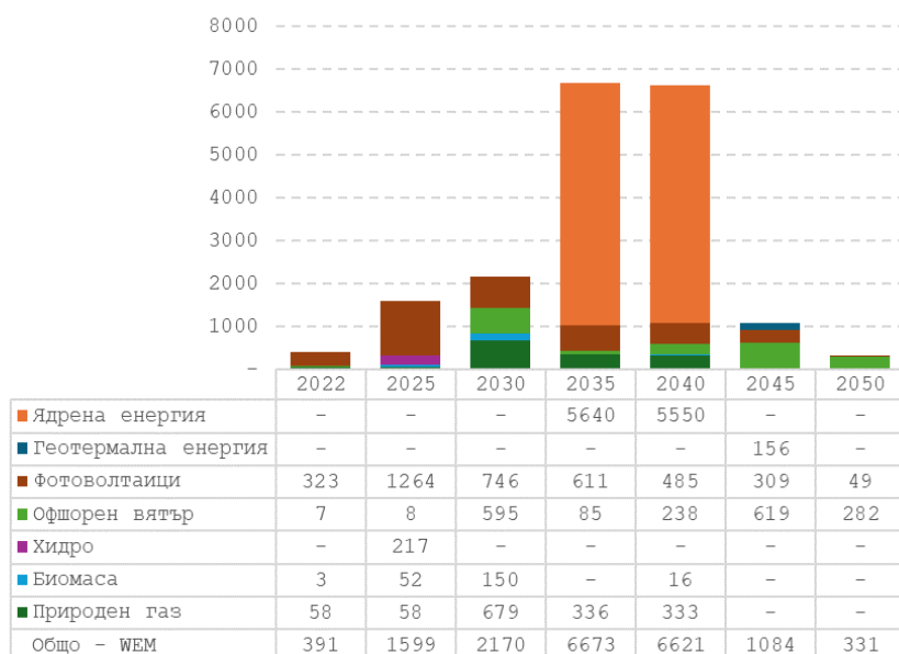
Фигура 121: Инвестиционни разходи за централите, произвеждащи електрическа енергия, (B)EST WEM прогнози (млн. EUR'15 за 5 год. период)
