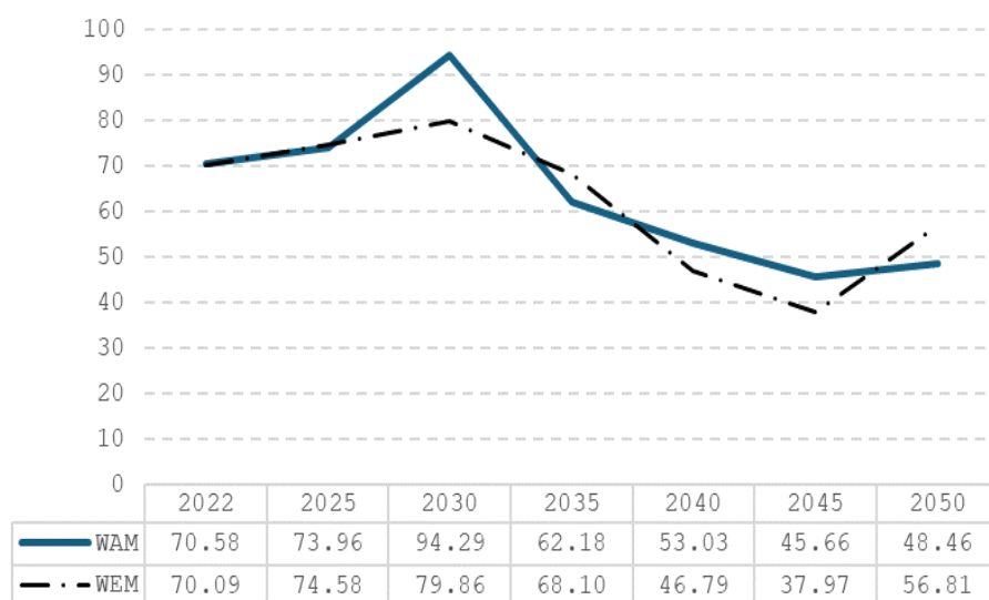
Фигура 102: Средни разходи за производство на електрическа енергия, исторически данни (2022 г.) и прогнози (B)EST WAM (2025-2050 г.), EUR'15/MWh
